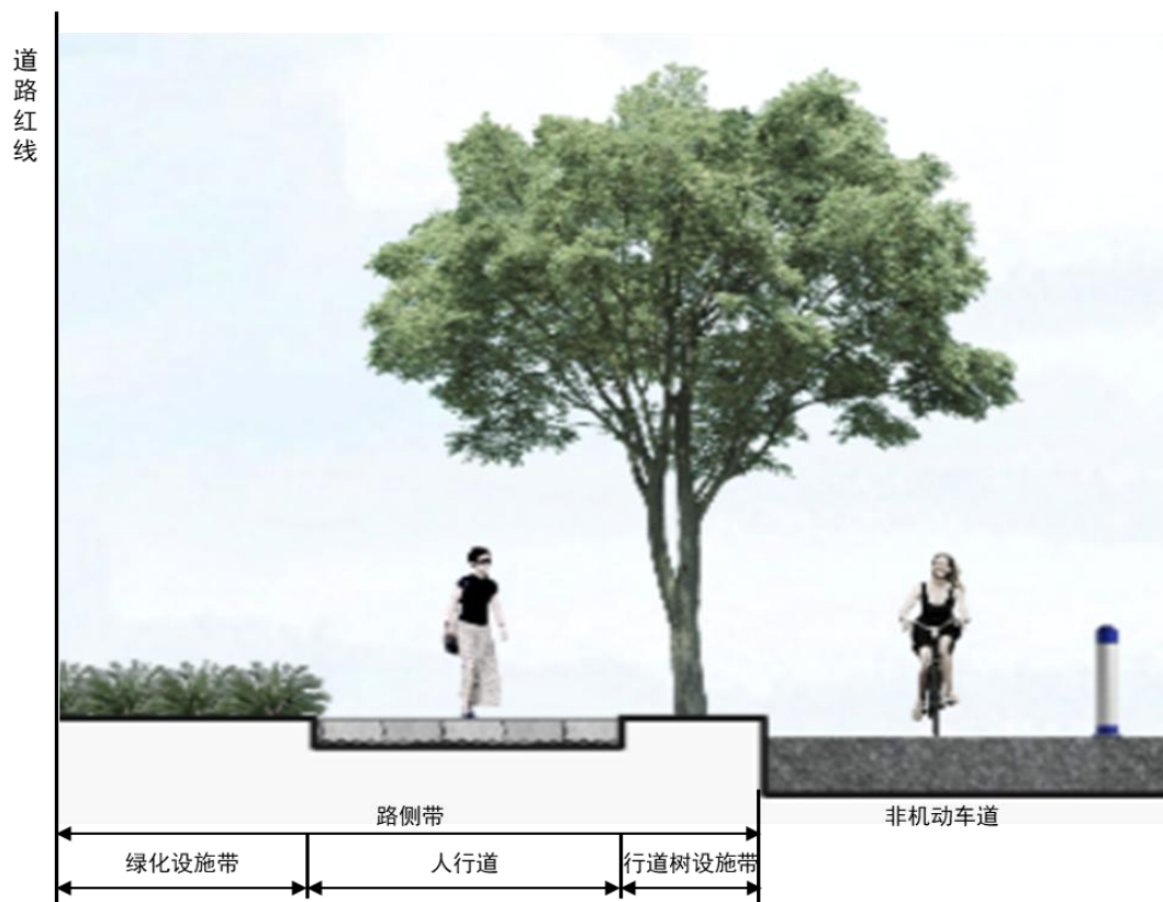
图 1 路侧带组成断面示意图
