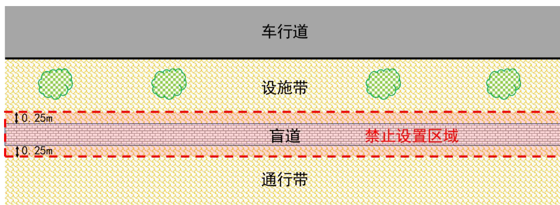
图 4 无障碍设施、盲道周边禁止设置区域示意图
