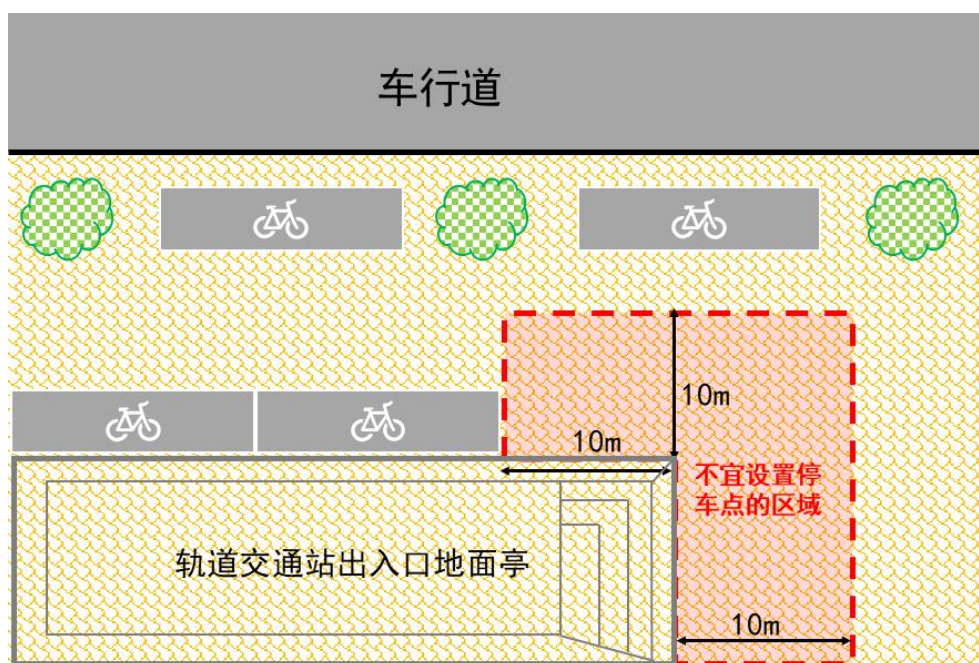
图 6 轨道交通站点出入口自行车停放区域设置示意图
