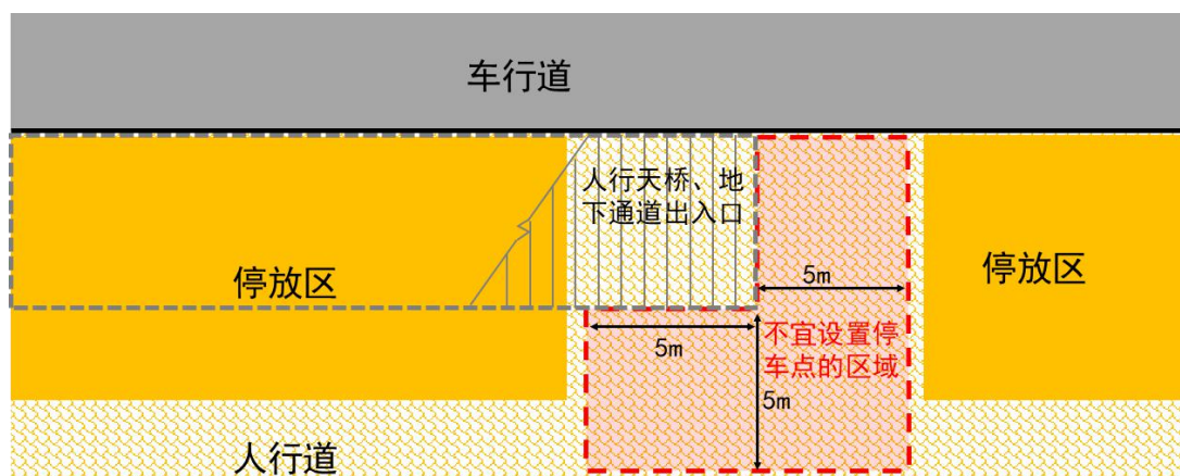
图9 人行天桥与地道出入口周边自行车停放区设置示意图
