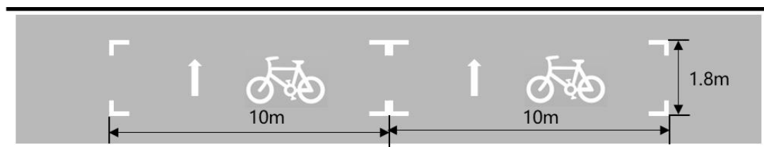
图 14 自行车停放区多组停放框示意图
