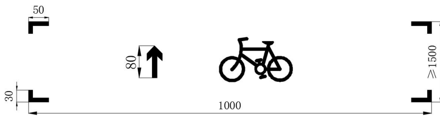
图 16 标线尺寸示意图（单位：cm）
