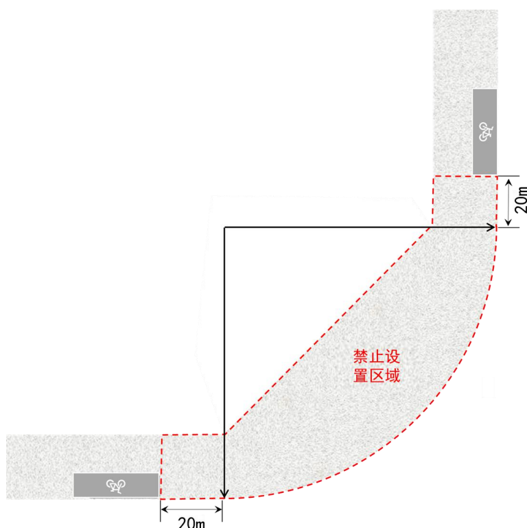
图 2 路口范围内禁止设置区域示意图
