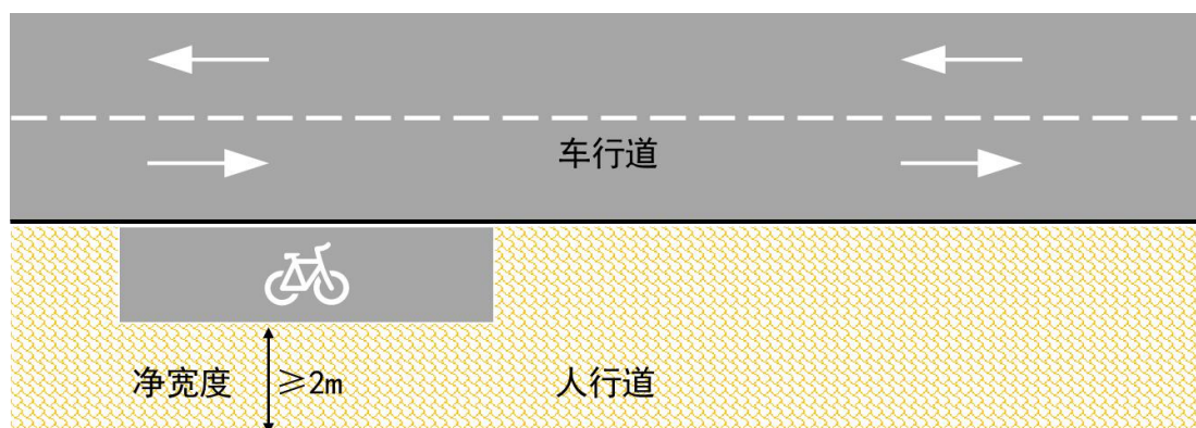
图 7 人行道剩余净宽度标准示意图
